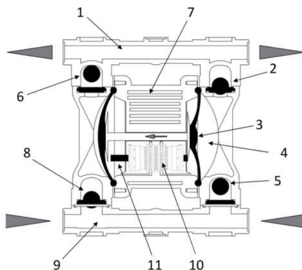
Рис. 2 : Конструкция насоса
